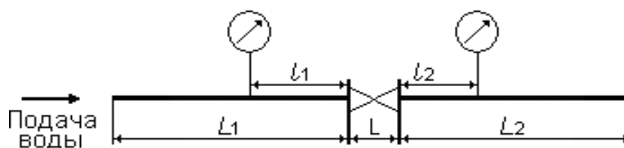
Рисунок 1 – Принципиальная схема участка испытательного стенда
